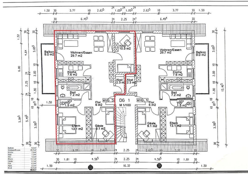
Grundrisse (Einzeichnung)
