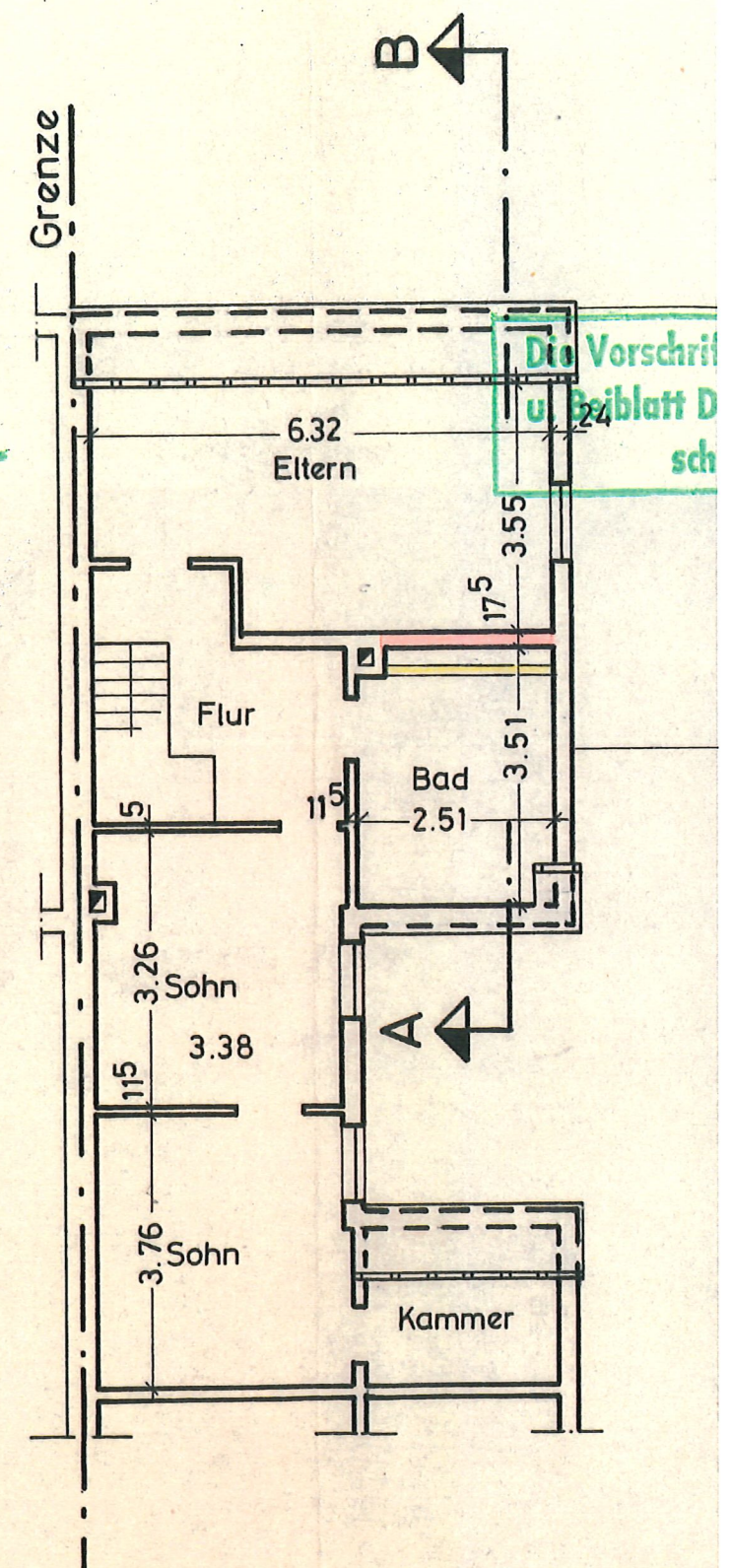
Dachgeschoß
