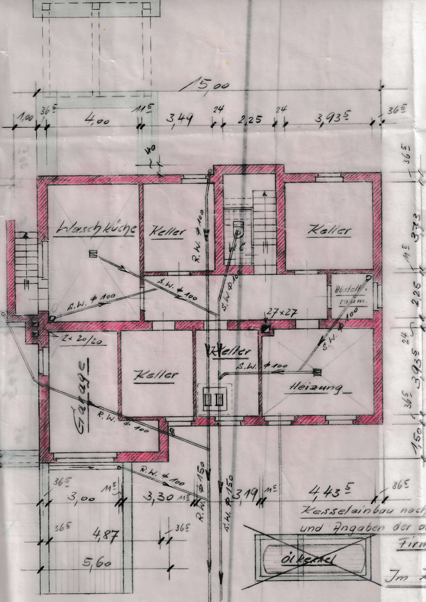
Kellergeschoss, M 1:100.
