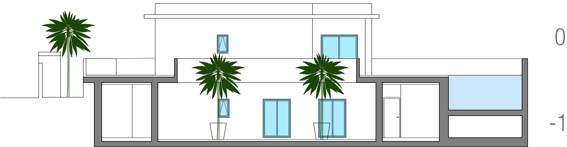
Façade B
