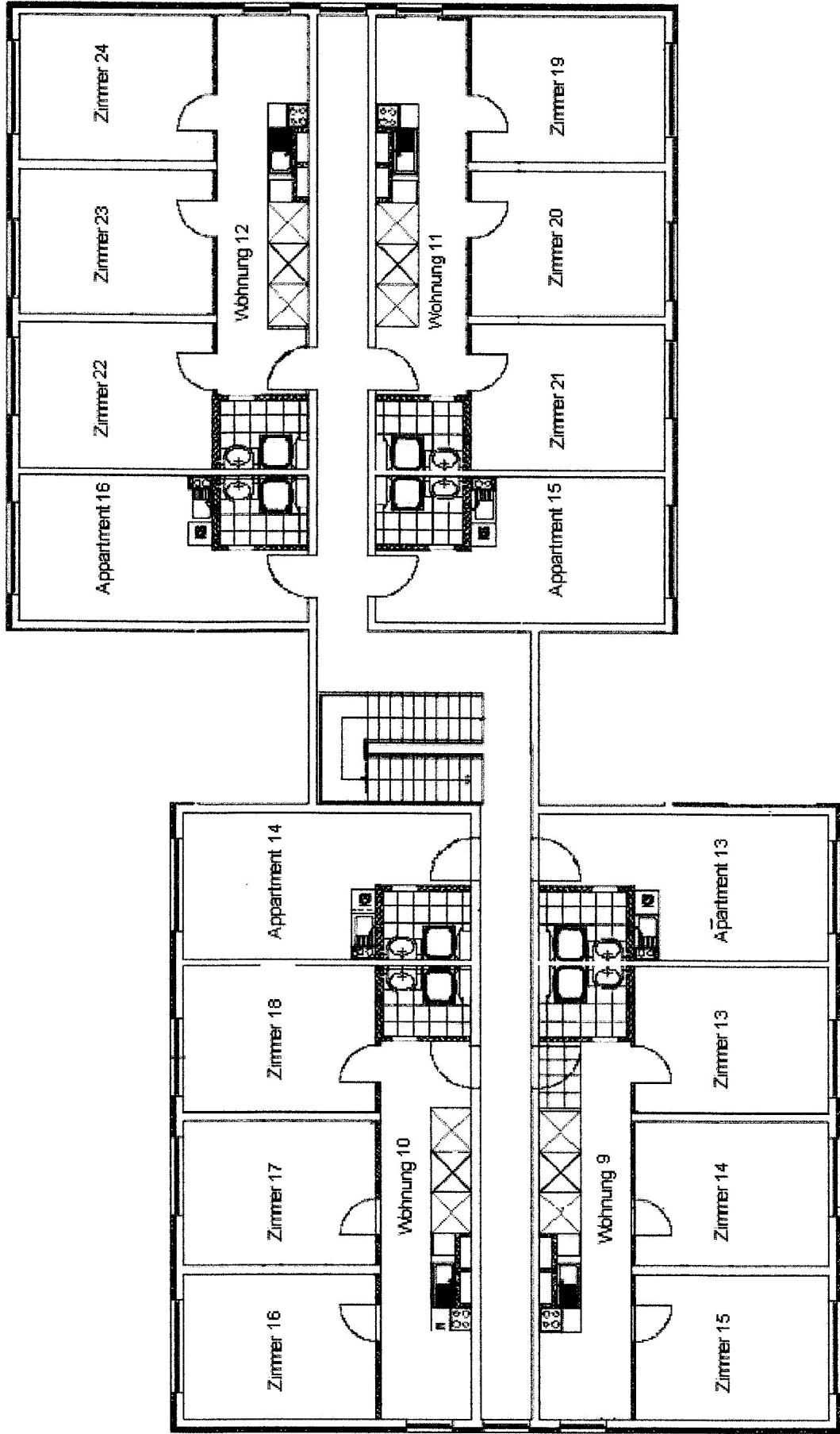
Grundriss 1. Obergeschoss
