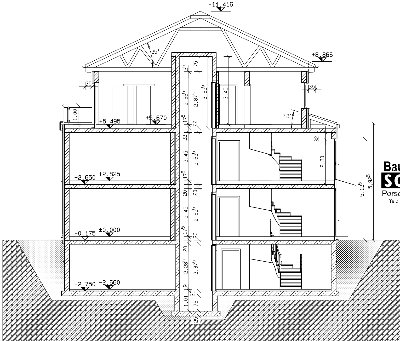
Schnitt A-A
