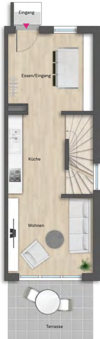
Erdgeschoss
