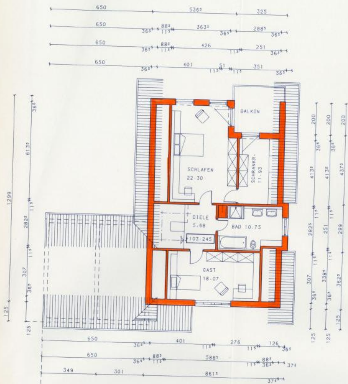
GRUNDRISS-DACHGESCHOSS
