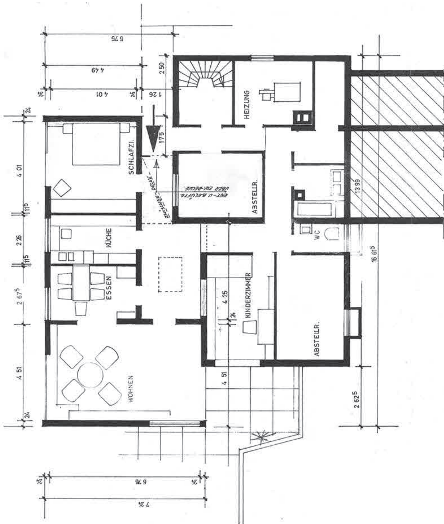
Wohnung 2
