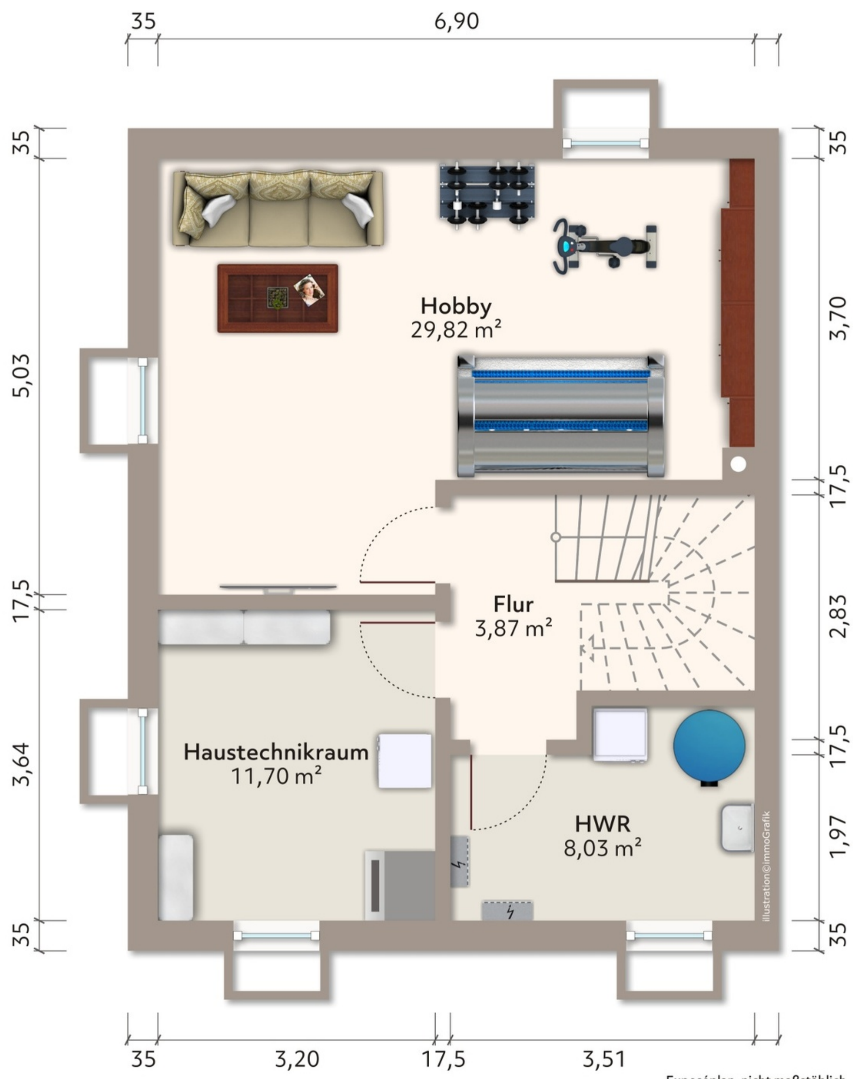
Exposéplan, nicht maßstäblich
