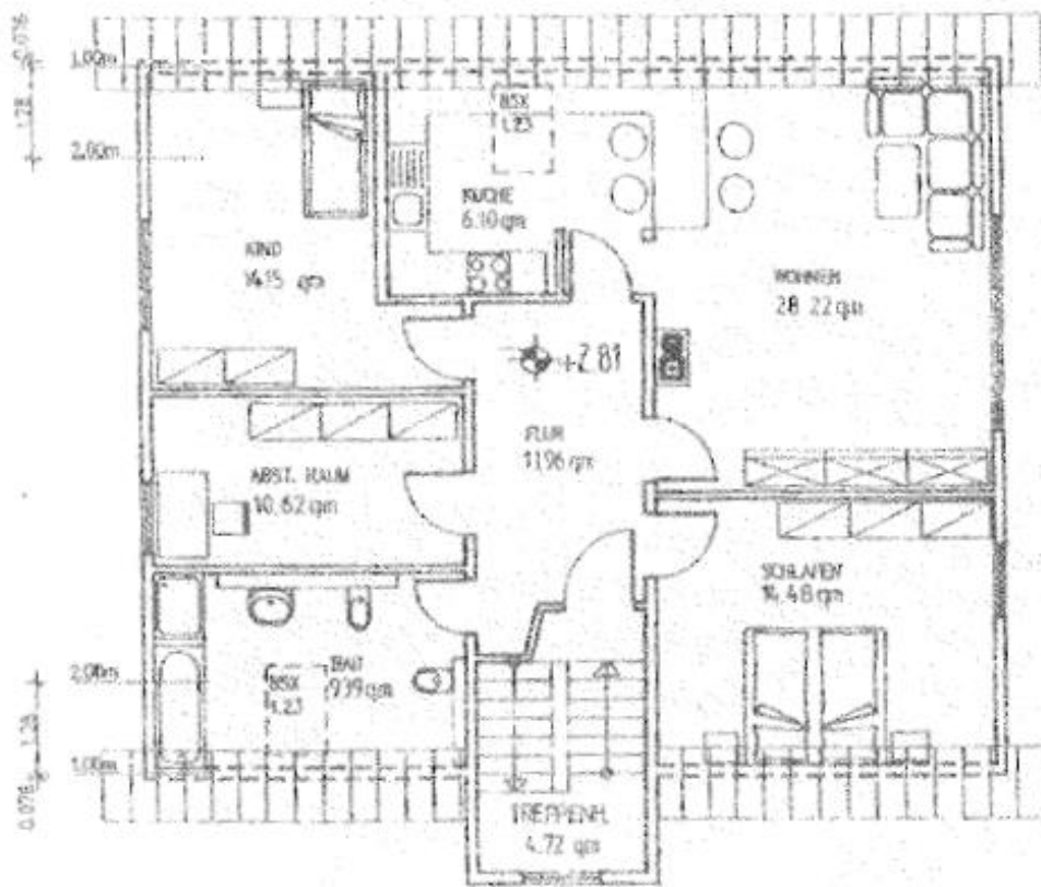
Grundriss Dachgeschoss
