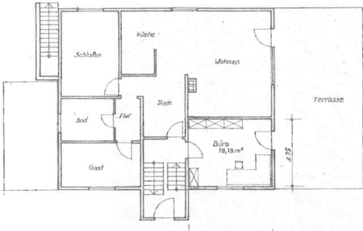
Grundriss Erdgeschoss
