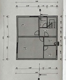
Grundriss KG
