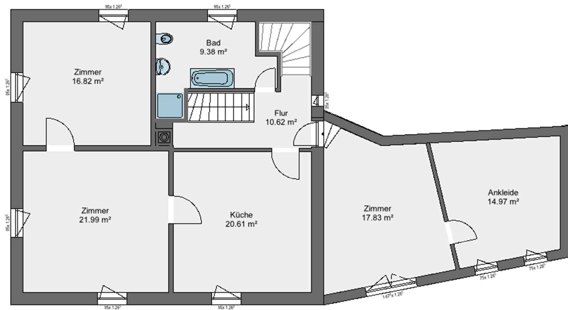
Grundriss - Obergeschoss - Steinstraße 49
