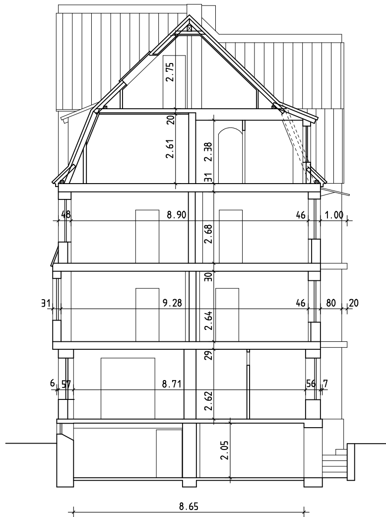
Schnitt B-B M 1:100
