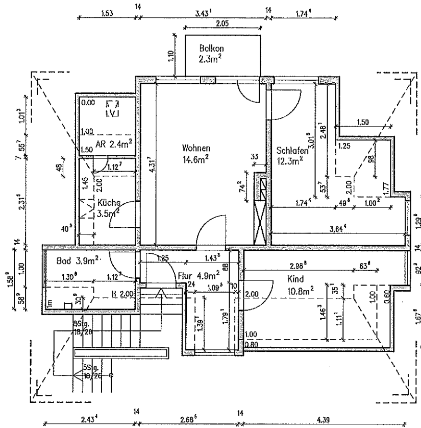
DACHGESCHOSS Flächenangaben im Plan sind Brutto-Geschoss-Flächen Die tatsächliche Wohnfläche siehe gesonderte Aufstellung.
