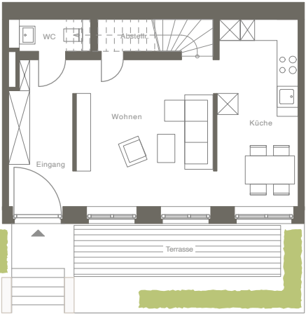
ERDGESCHOSS
