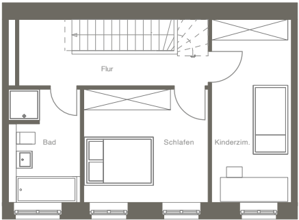
1. OBERGESCHOSS
