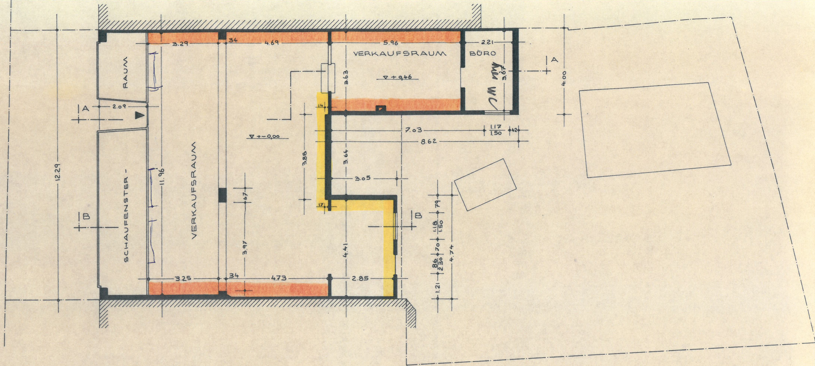
ERDGESCHOSS - GRUNDRISS
