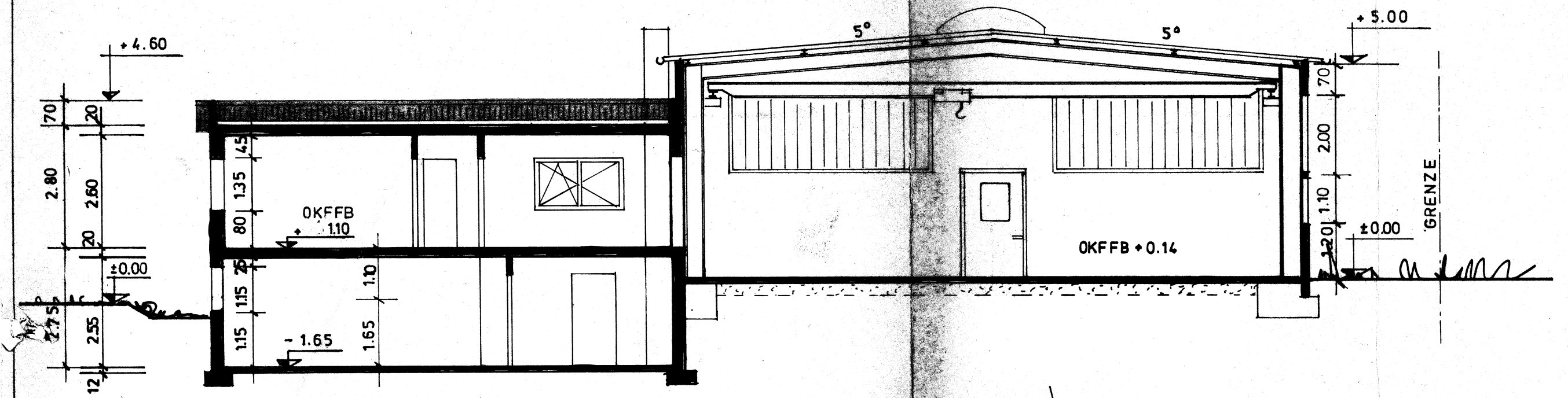
SCHNITT A-A
