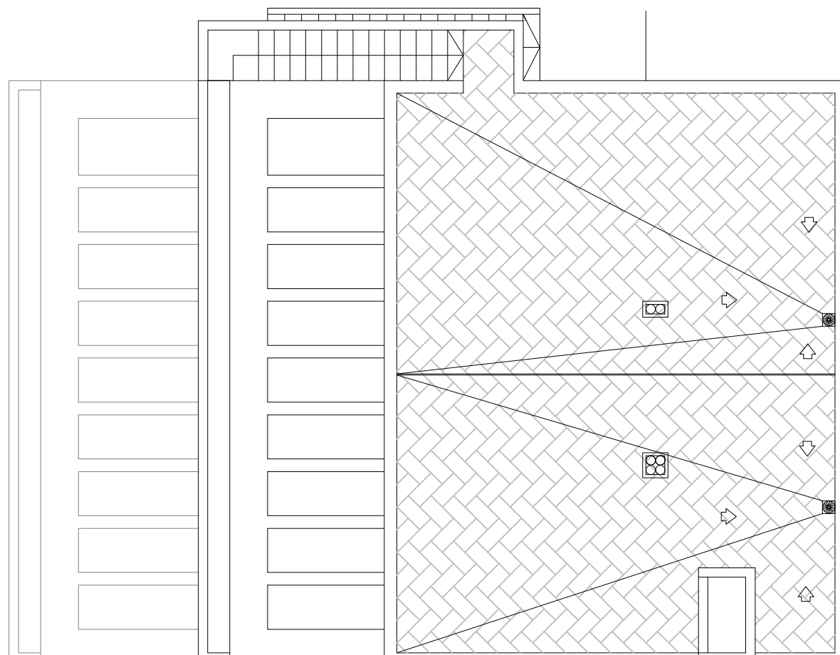
Planta Solarium
