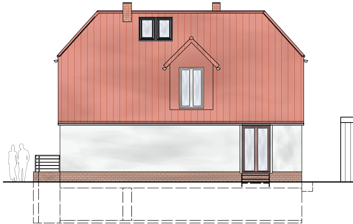
ANSICHT NORD
