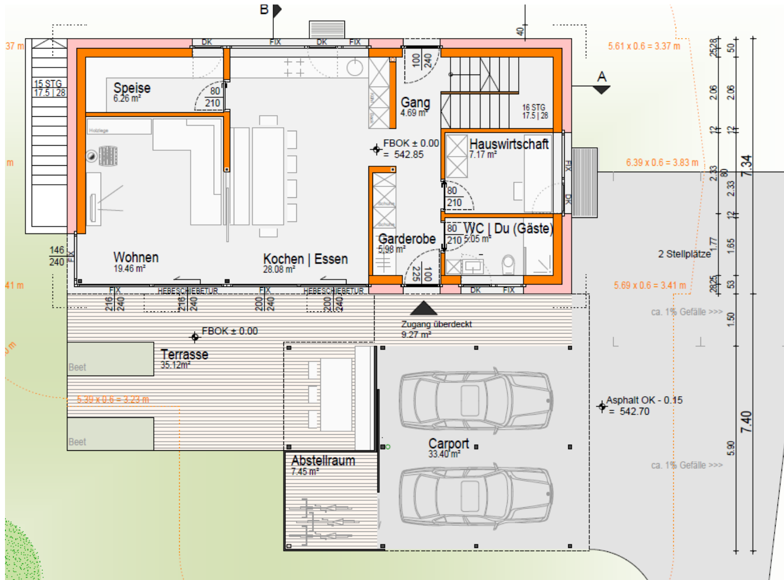
Plan EG
