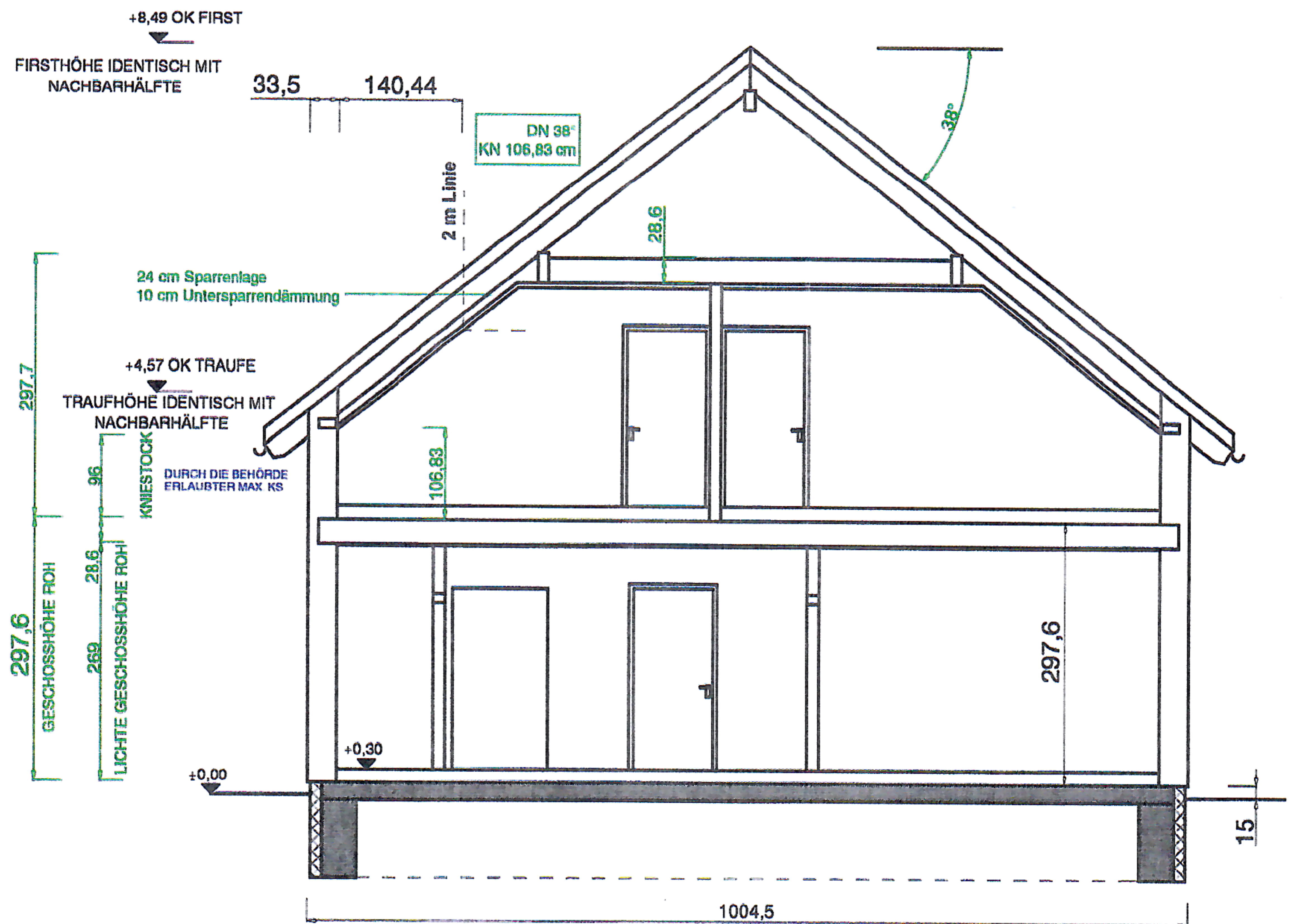
SCHNITT A - A m 1:100
