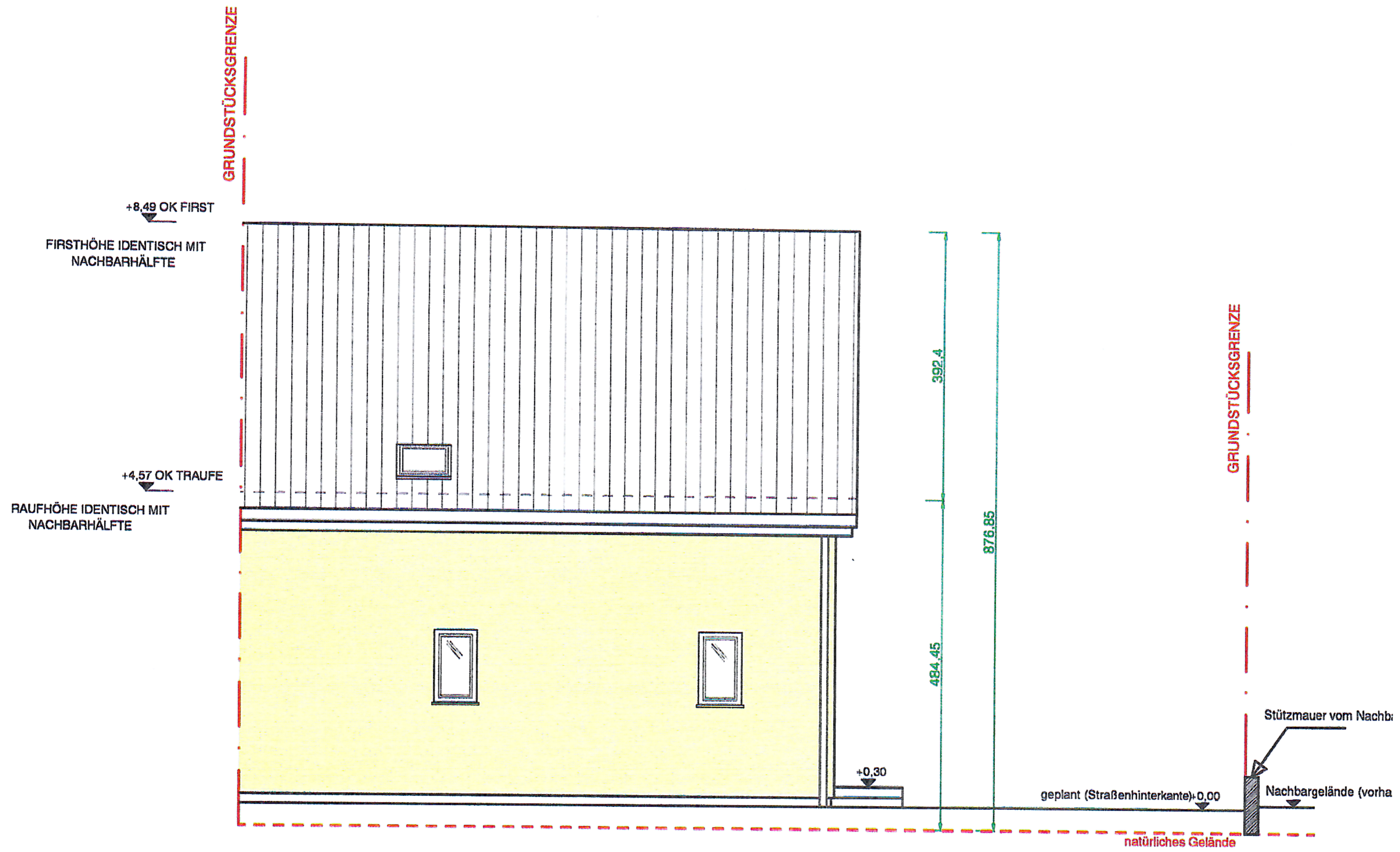
NORDANSICHT m 1:100
