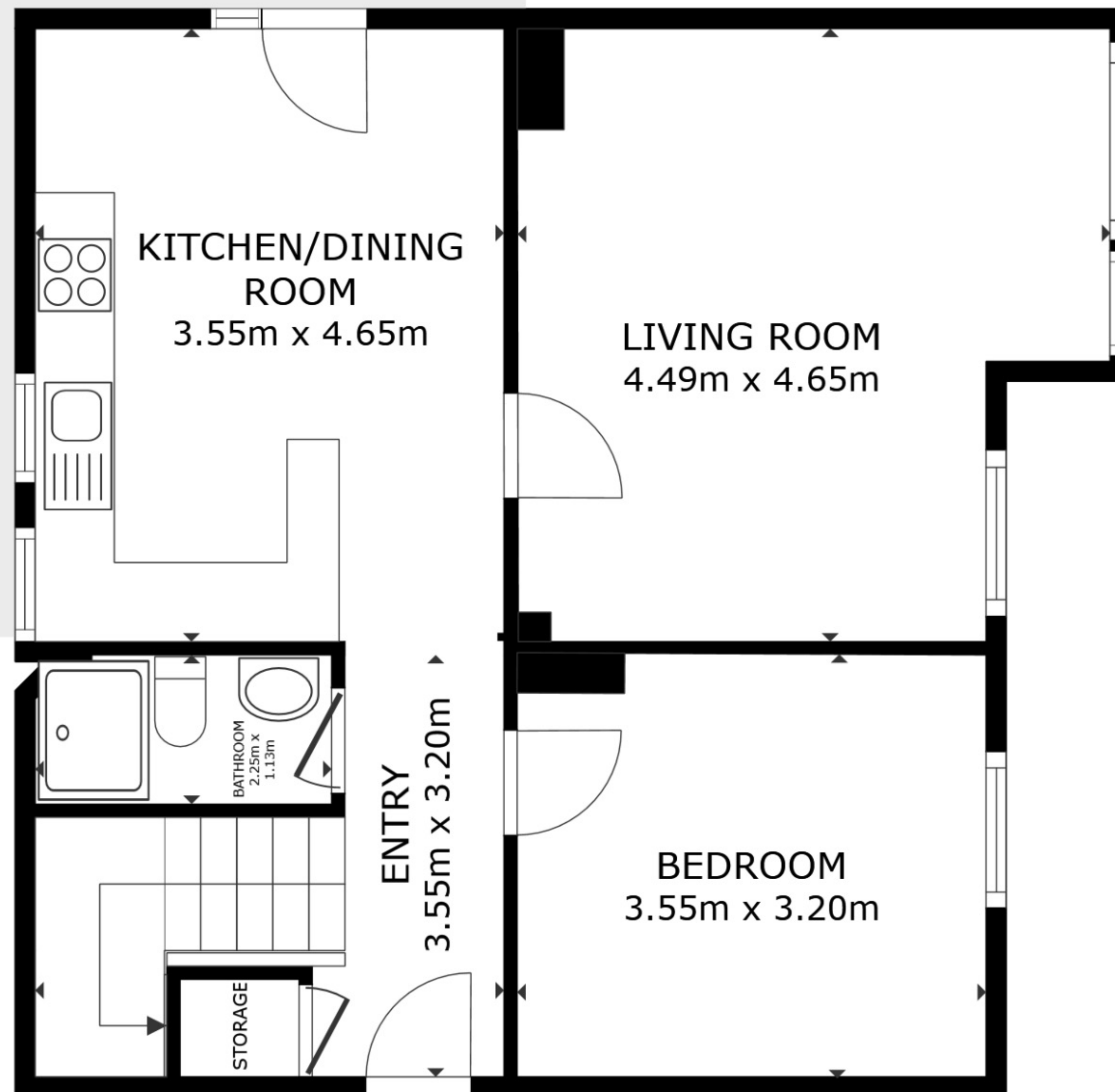
ERDGESCHOSS
