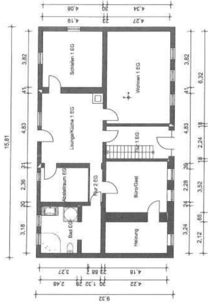
Grußendorf Immobilien & Finanzdienste Erdgeschoss Maßstab 1:100
