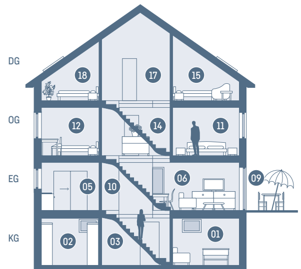
Schnitt 1:200
