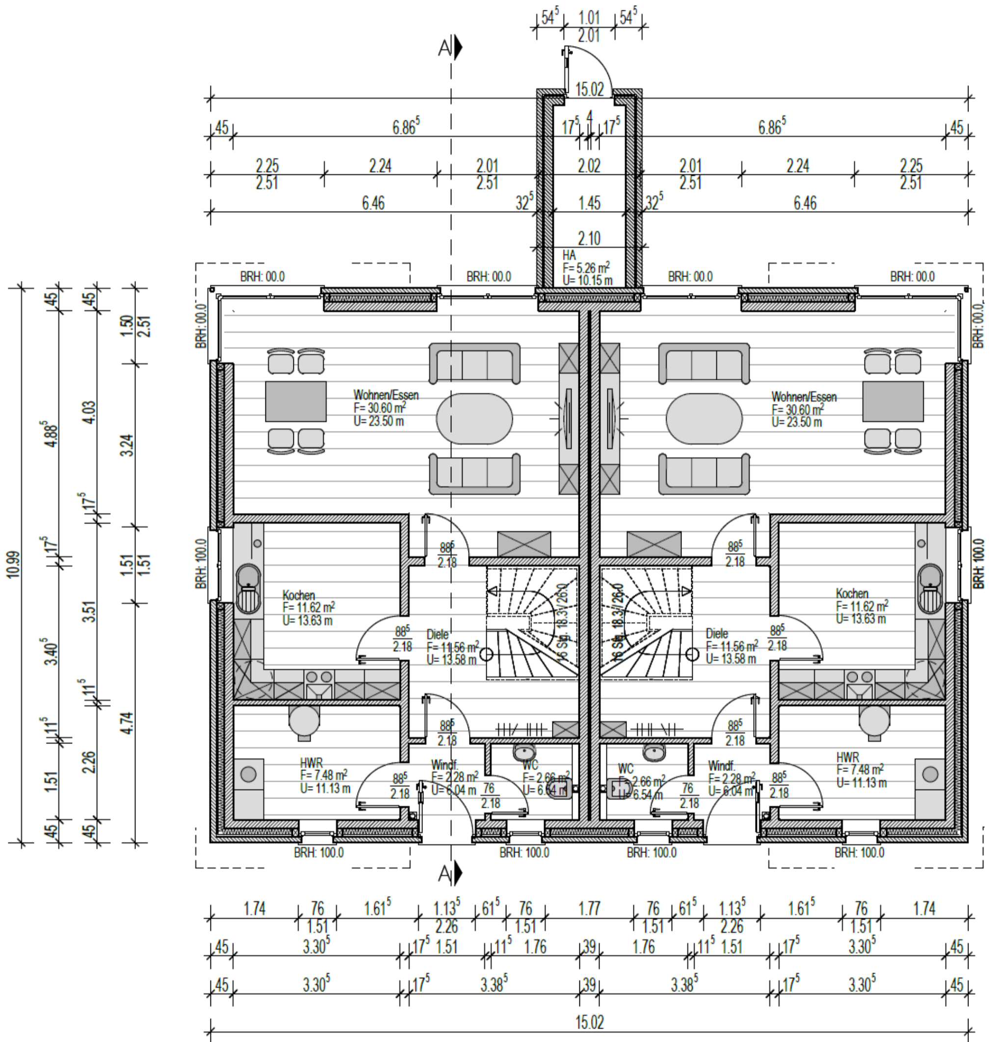
Erdgeschoss-Grundriss
