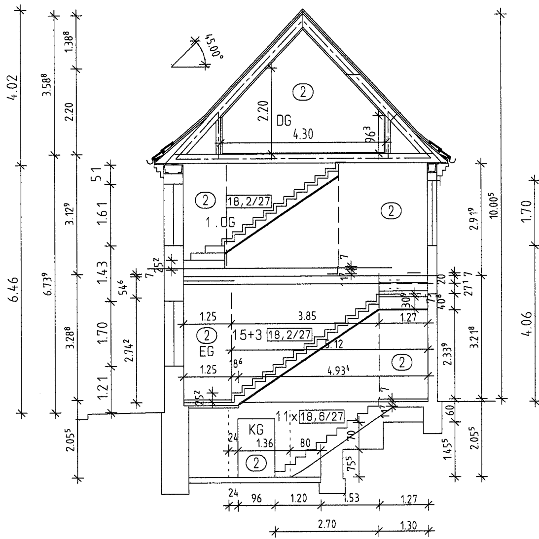
Gebäudeschnitt (A-A)
