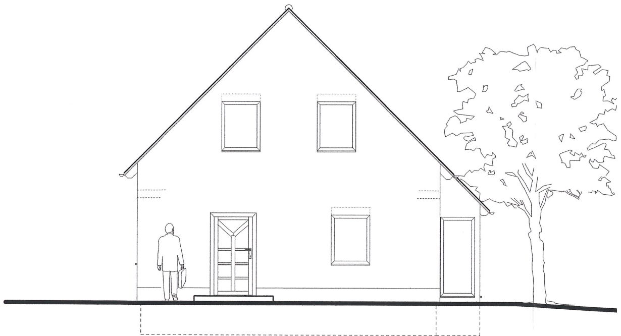
ANSICHT NORD
