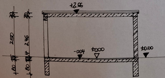
Schnitt B-B
