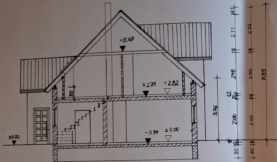
Schnitt A-A
