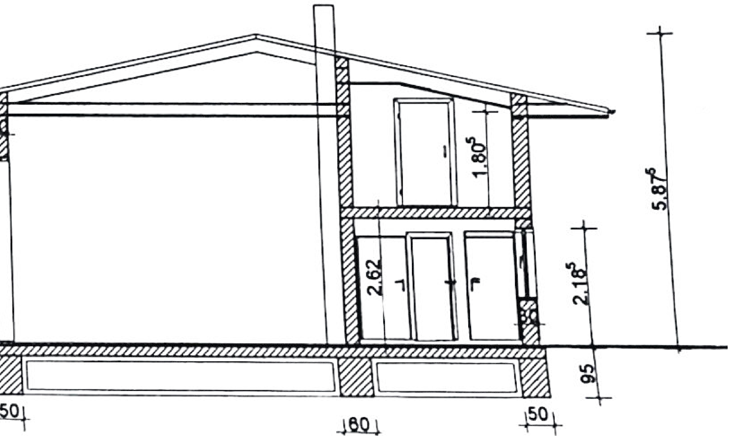
Hallenquerschnitt
