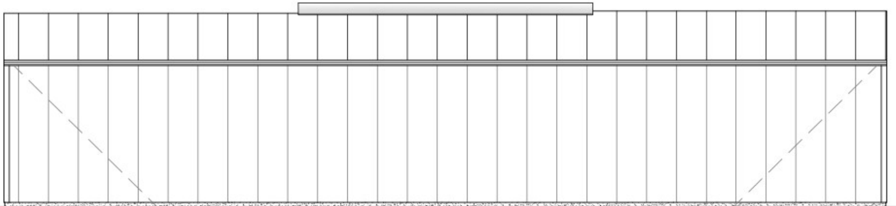
Nordwestansicht (Achse A)
