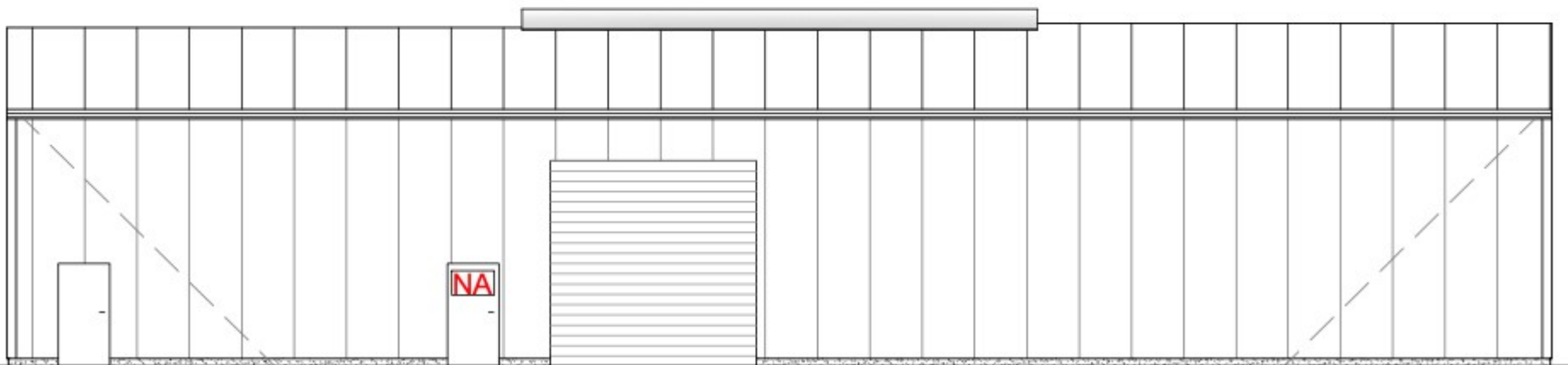
Südostansicht (Achse B)
