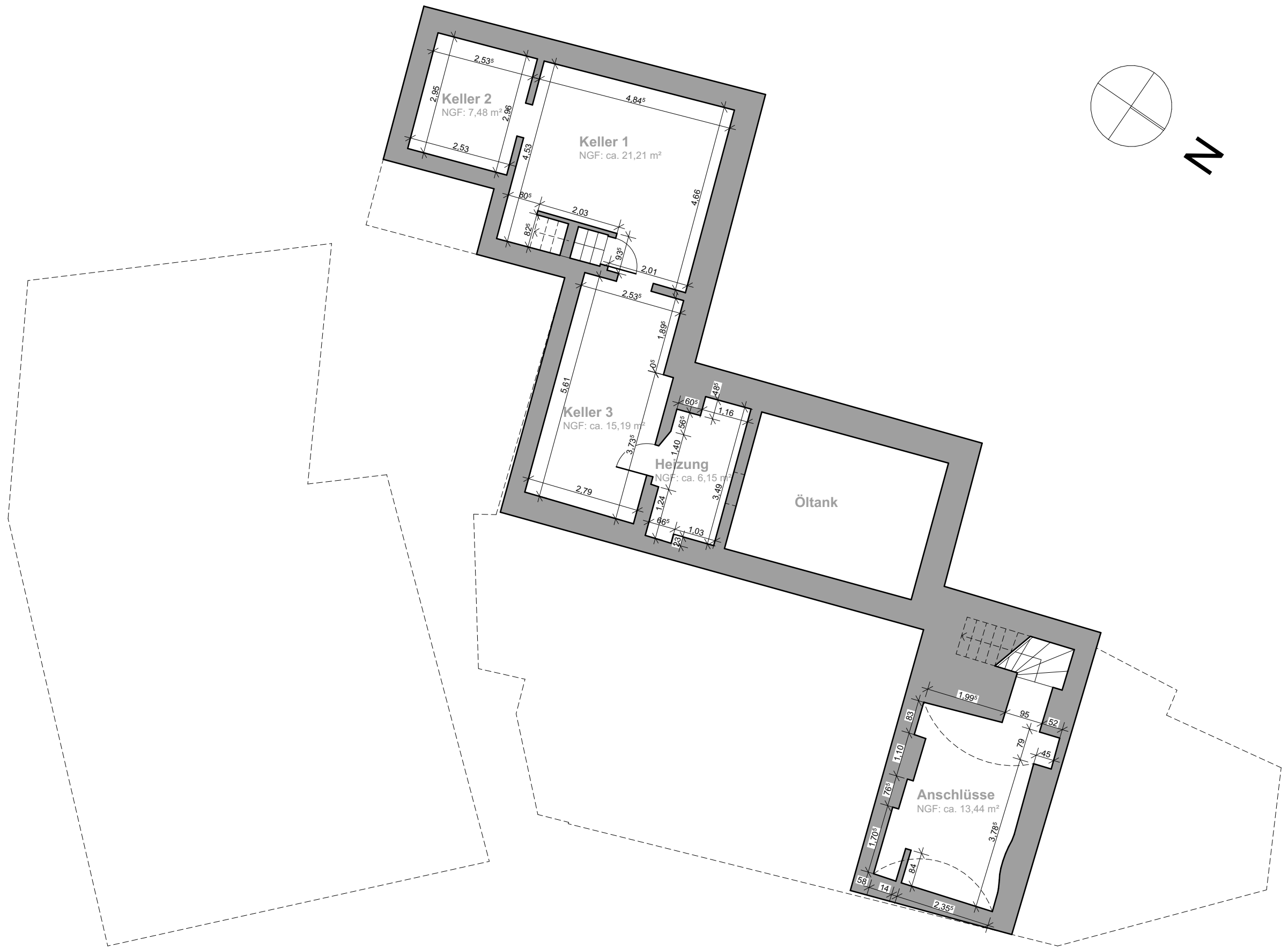
Grundriss KG
