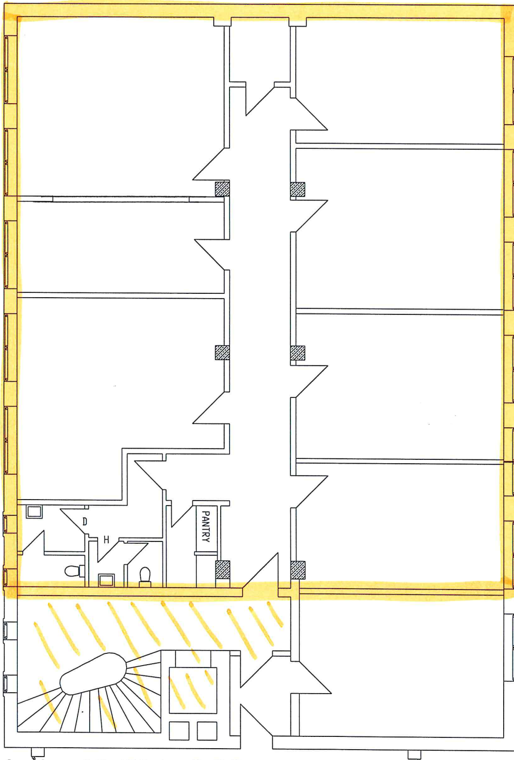
Ausbau Mietfläche 2 OG. Gotenstr.19 , 20097 Hamburg M=ca 1:100
