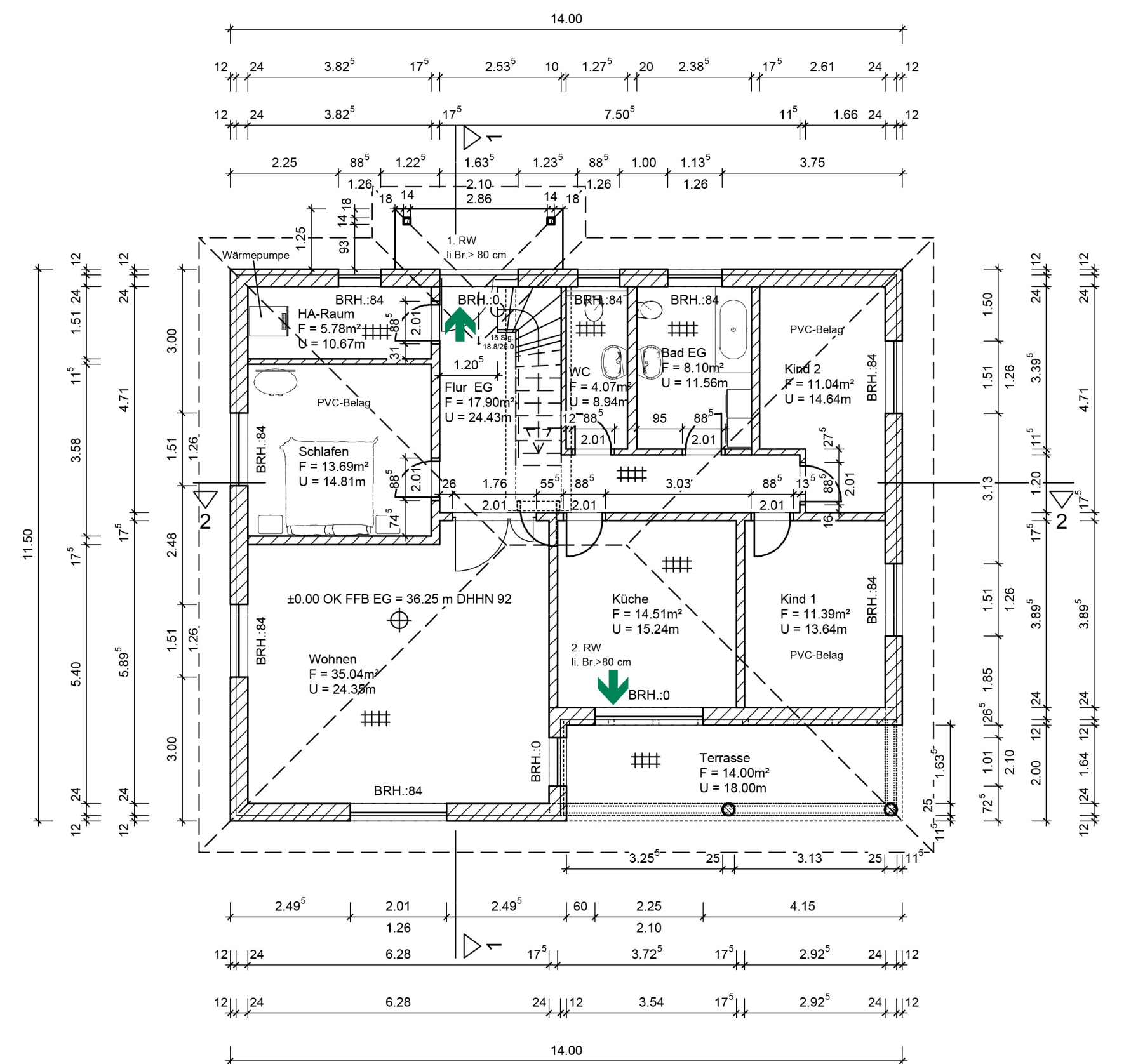
Grundriss Erdgeschoss (WHS)
