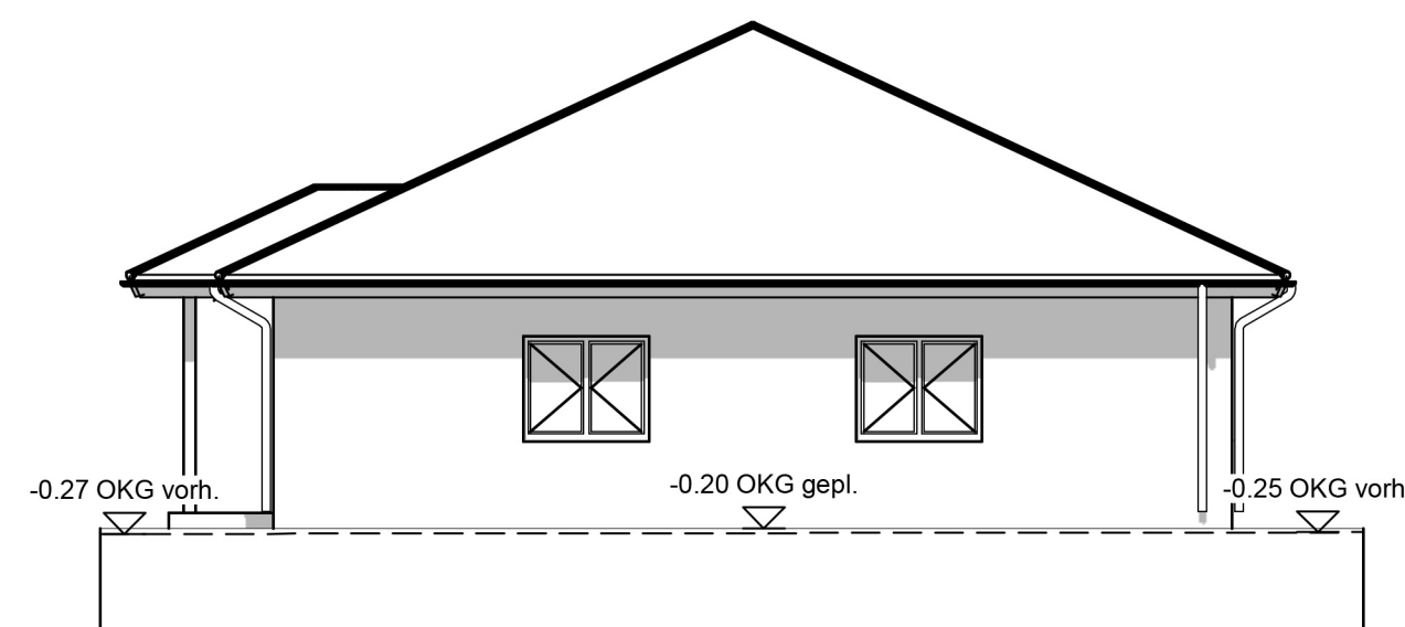
NW-Ansicht (WHS)
