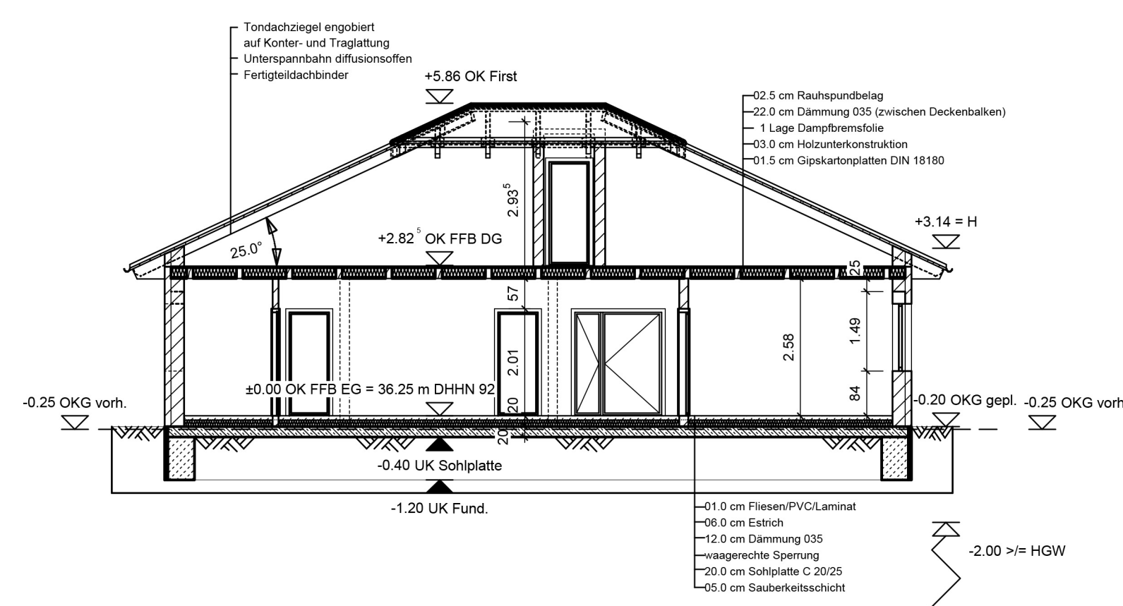
Schnitt 2 - 2 (WHS)
