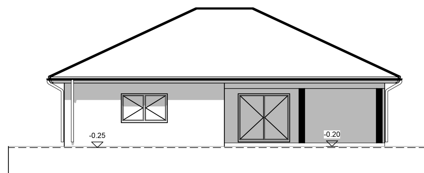
SW-Ansicht (WHS)
