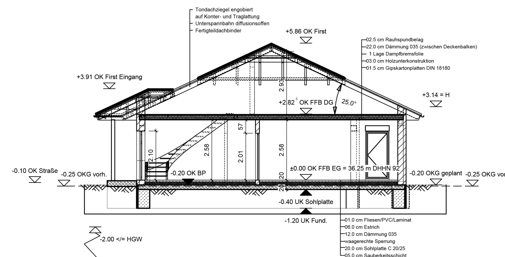
Schnitt 1 - 1 (WHS)
