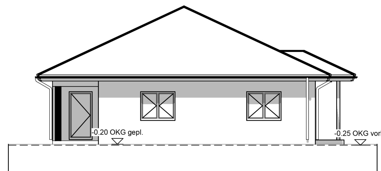
SO-Ansicht (WHS)
