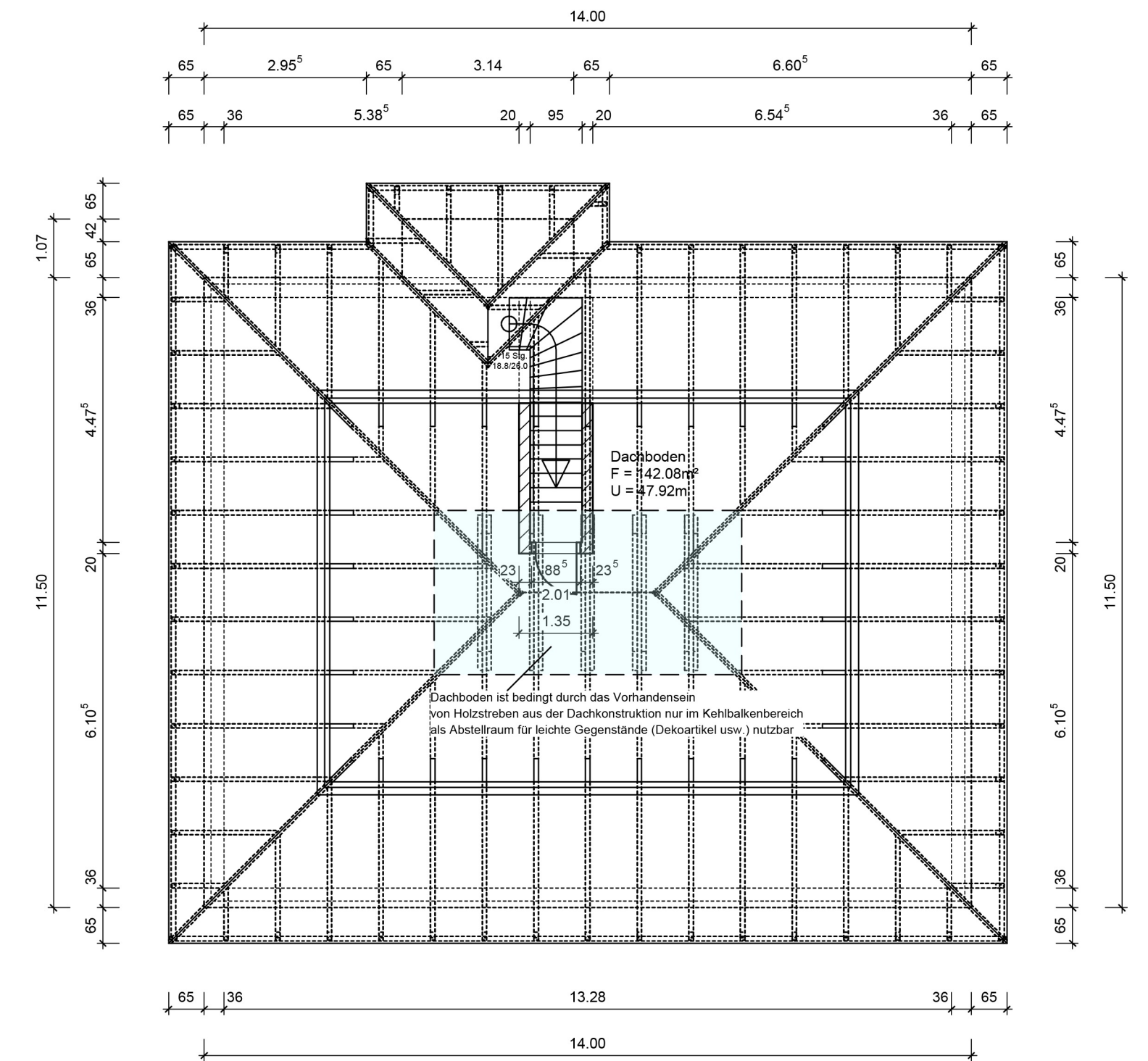
Grundriss Dachgeschoss (WHS)
