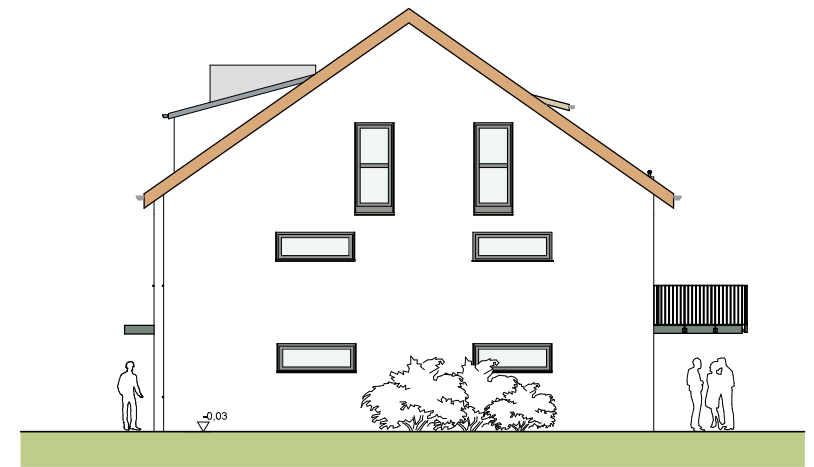
Ansicht Westen
