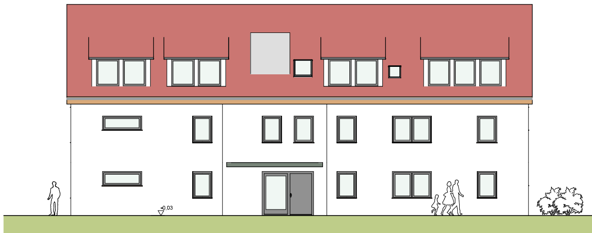
Ansicht Norden
