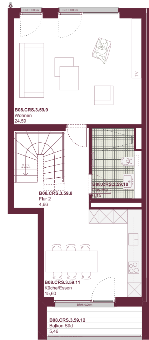
Grundriss 3. Obergeschoss M 1:100
