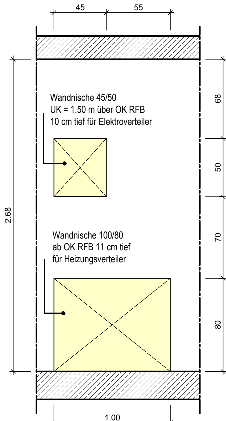
Detail- Regelschnitt Wandnischen für Wohnungsverteilung (Heizung und Elektro) M 1:20
