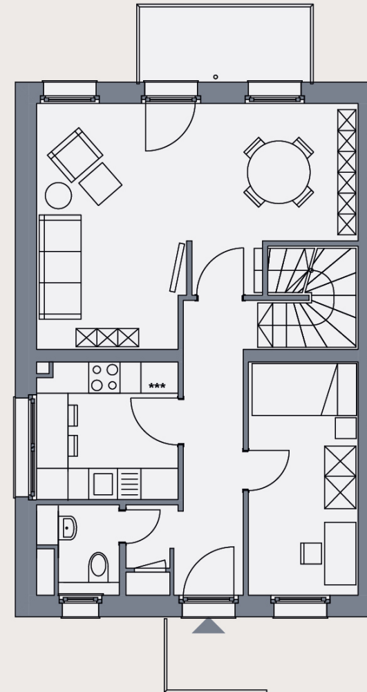
ERDGESCHOSS
