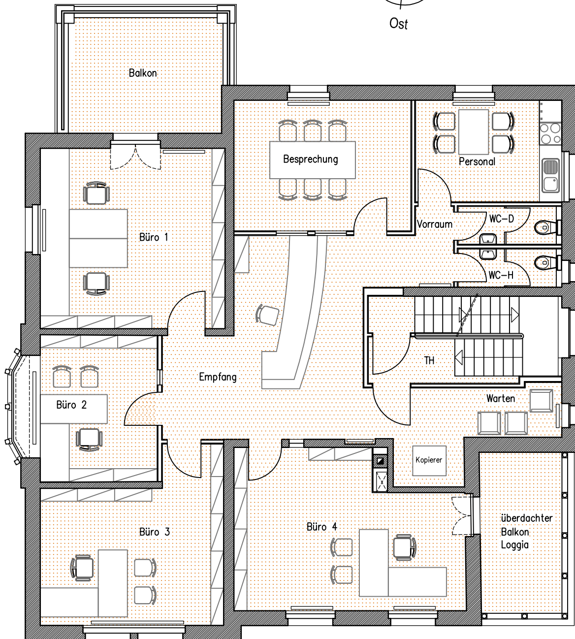
1. Obergeschoss
