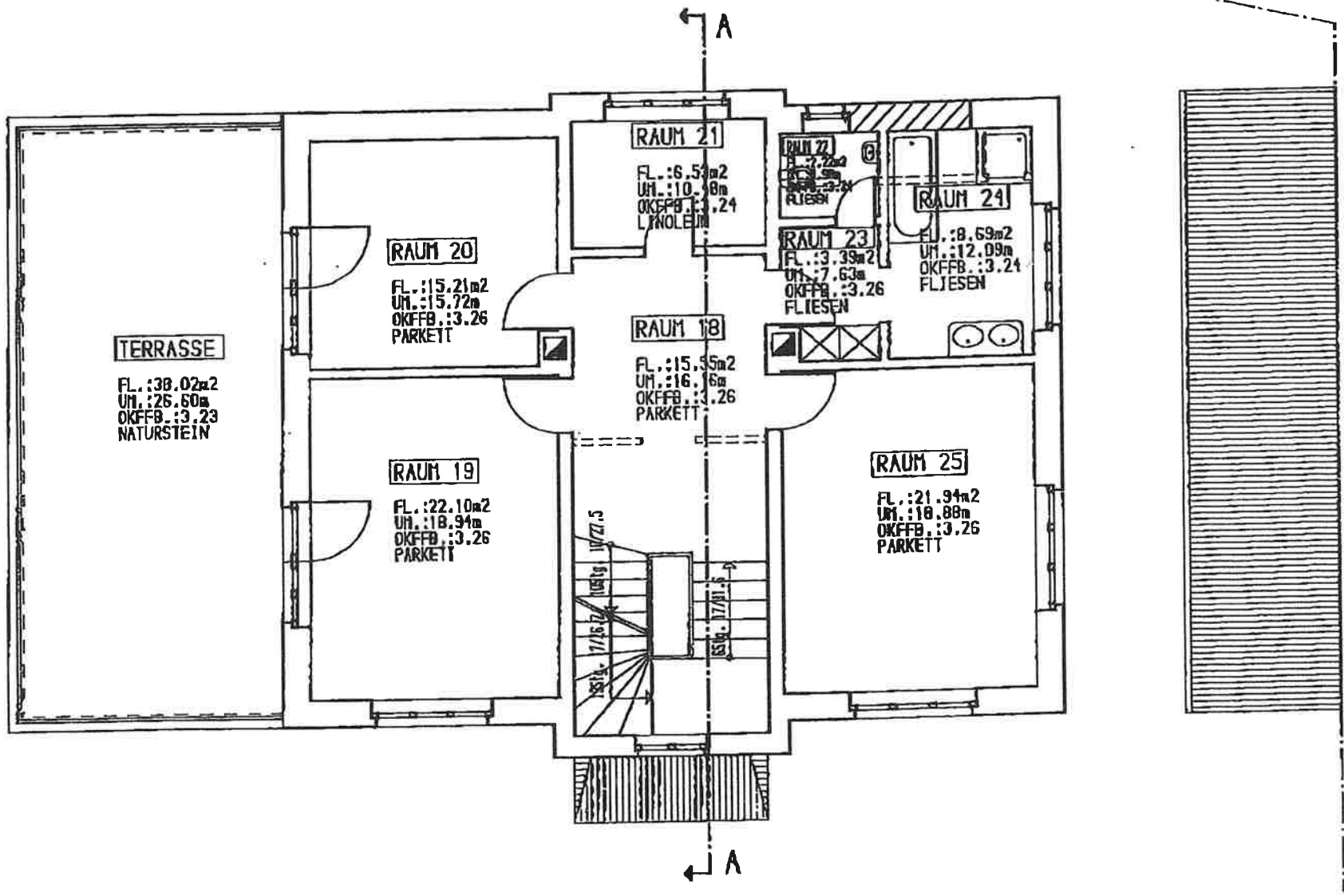
OBERGESCHOSS M:1/100
