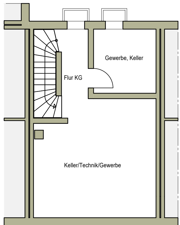
Kellergeschoss
