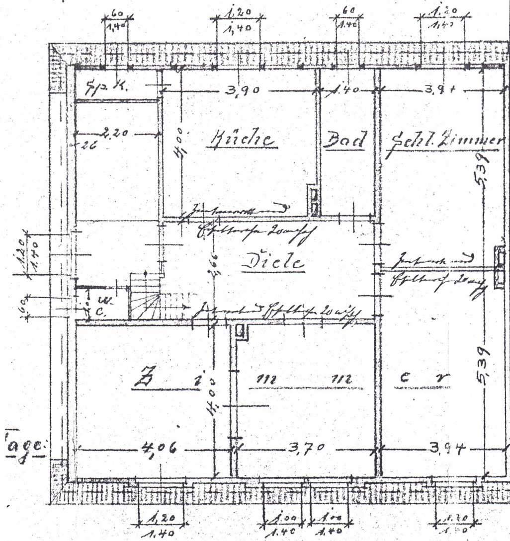
II. Obergeschoss
