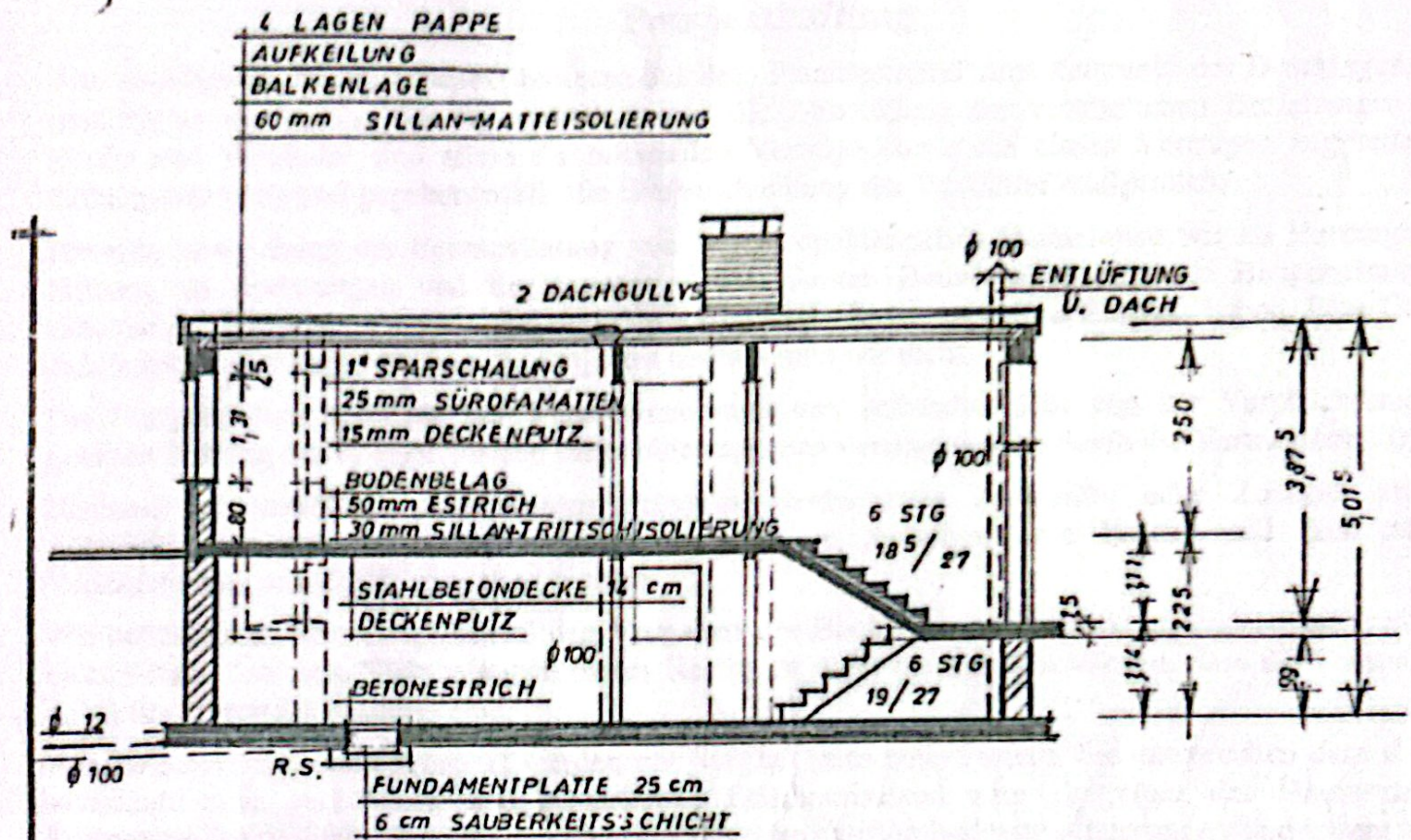
SCHNITT A-B
