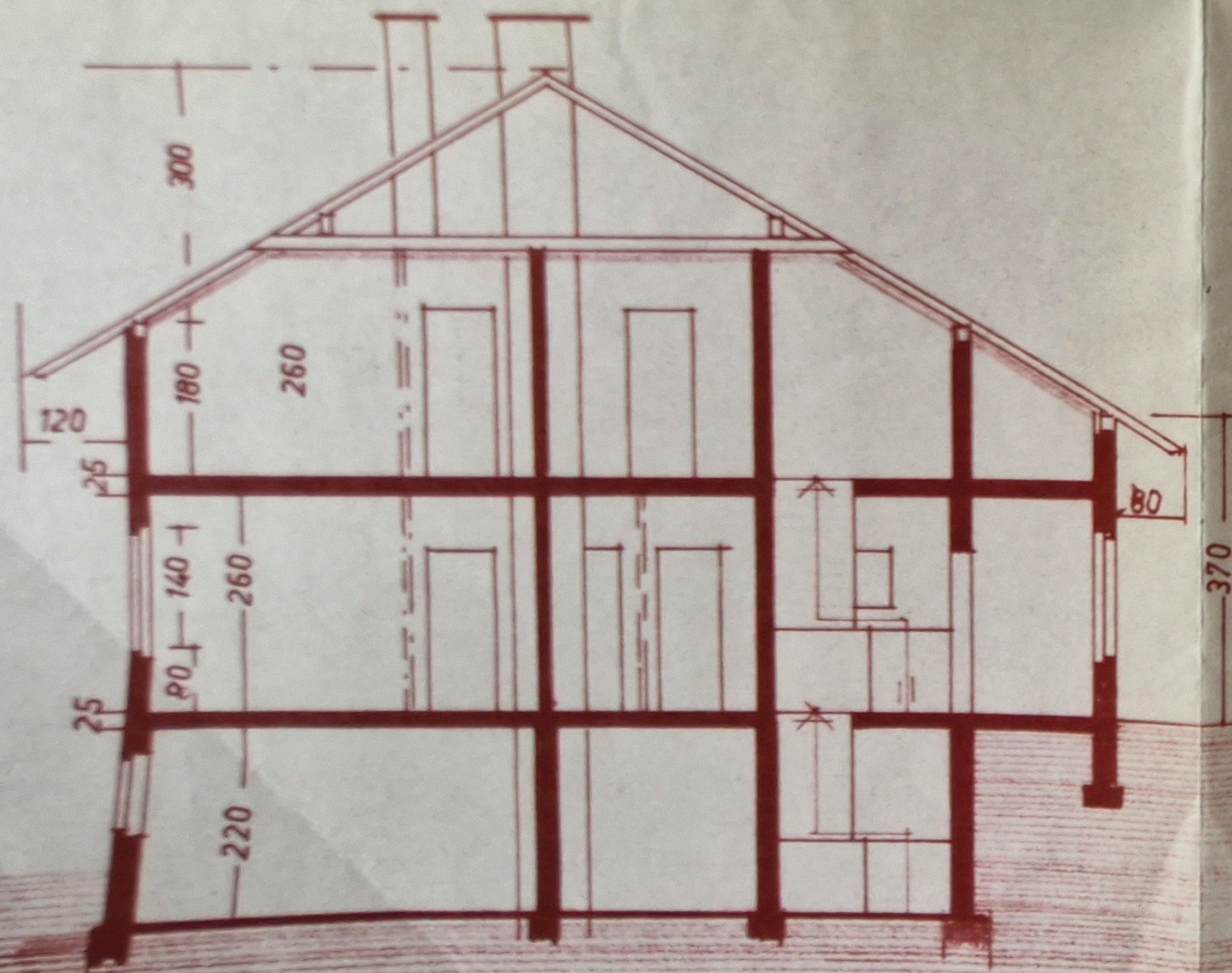
Schnitt: A-B
