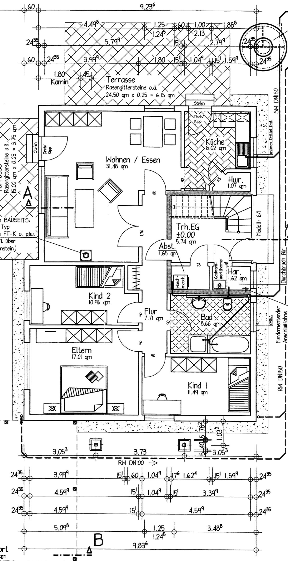
Erdgeschoss ■ Wohnungstrennwand (Schallschutzwand)
