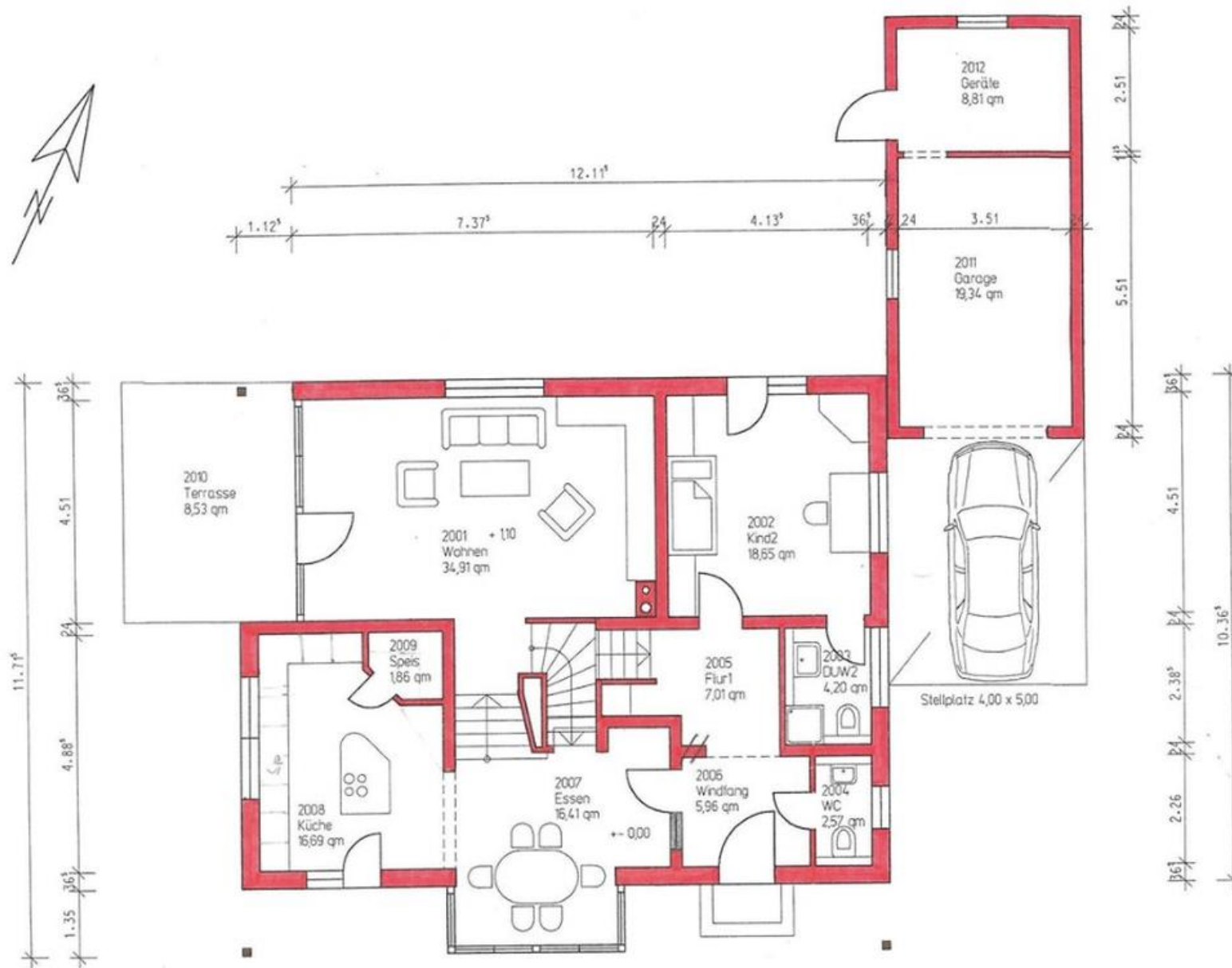
Erdgeschoss
