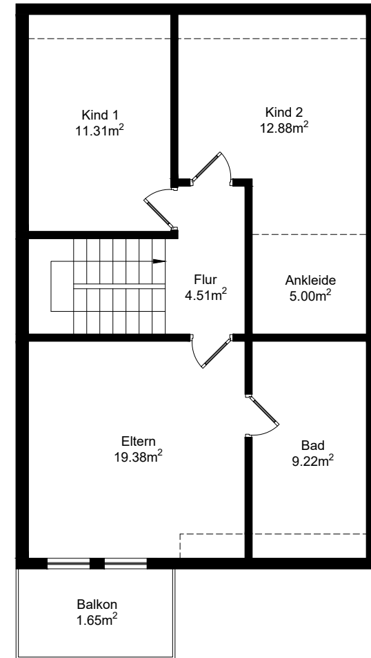
Obergeschoss 2
