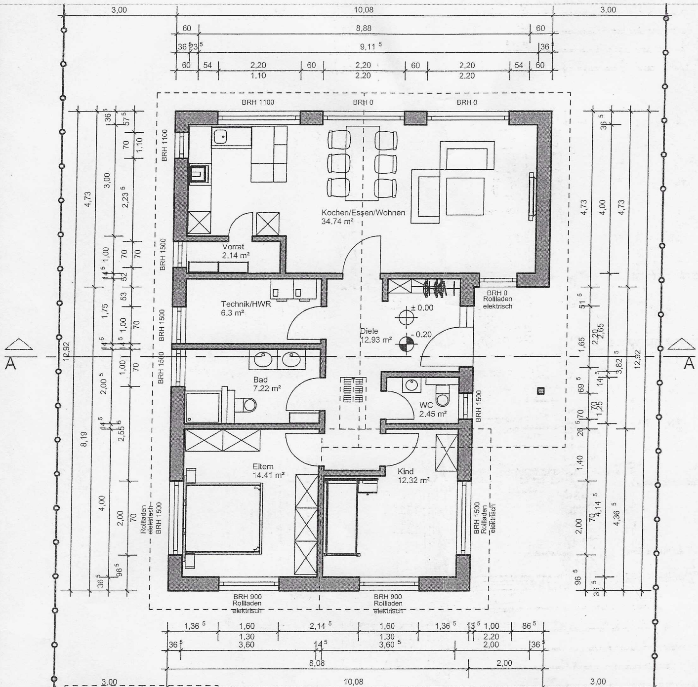
Grundriss Erdgeschoss
