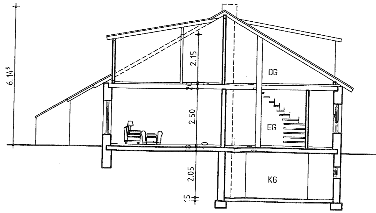
Schnitt
