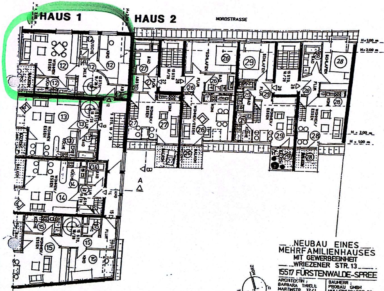
1. DACHGESCHOSS
